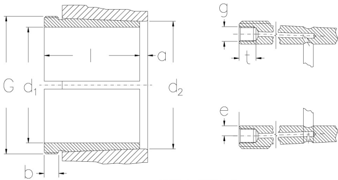
AOH(X) & AOH(X) .. G Kegel 1:12 (Kegel 1:30 bei H240, H241)
